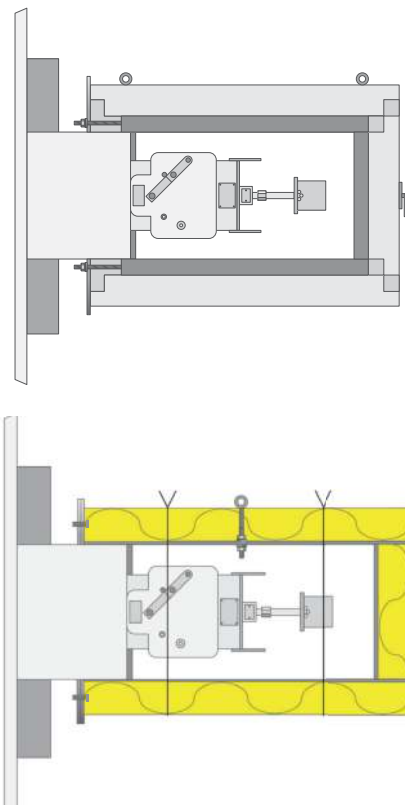
Box antincendio DS STOP FIRE su densimetro
