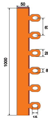
MT spessore 50 mm taglio in cantiere
